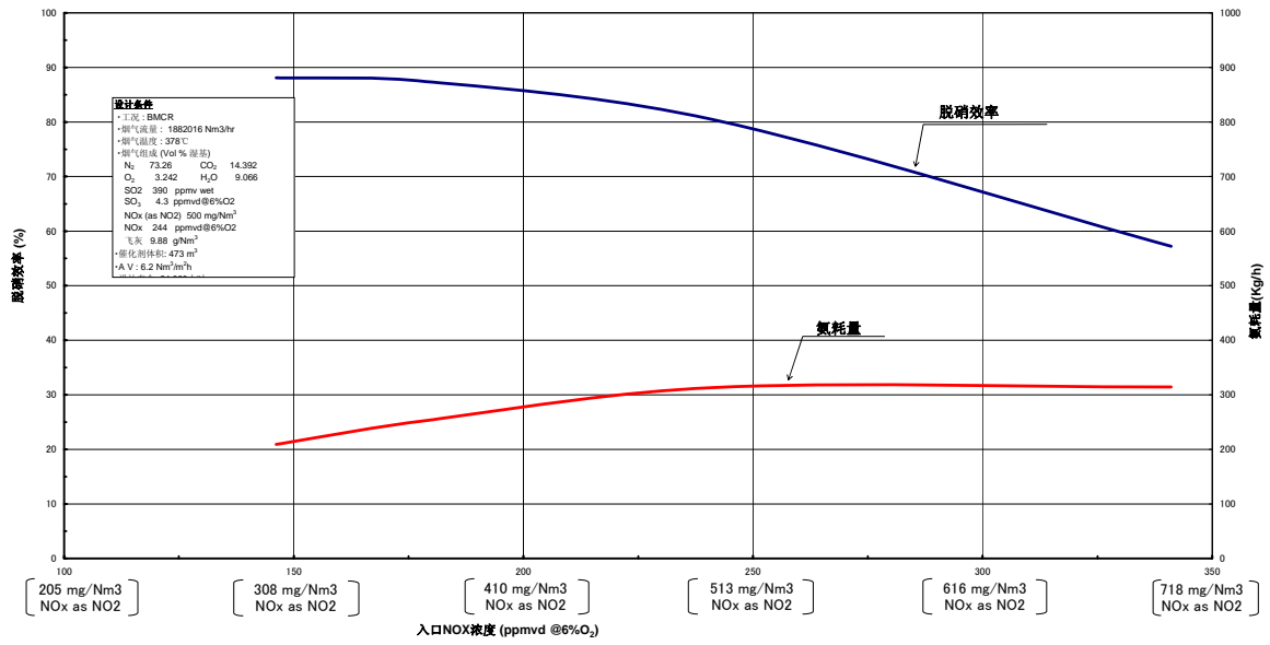
图 D.3 脱硝效率（氨耗量）与入口 NO x 浓度的关系
