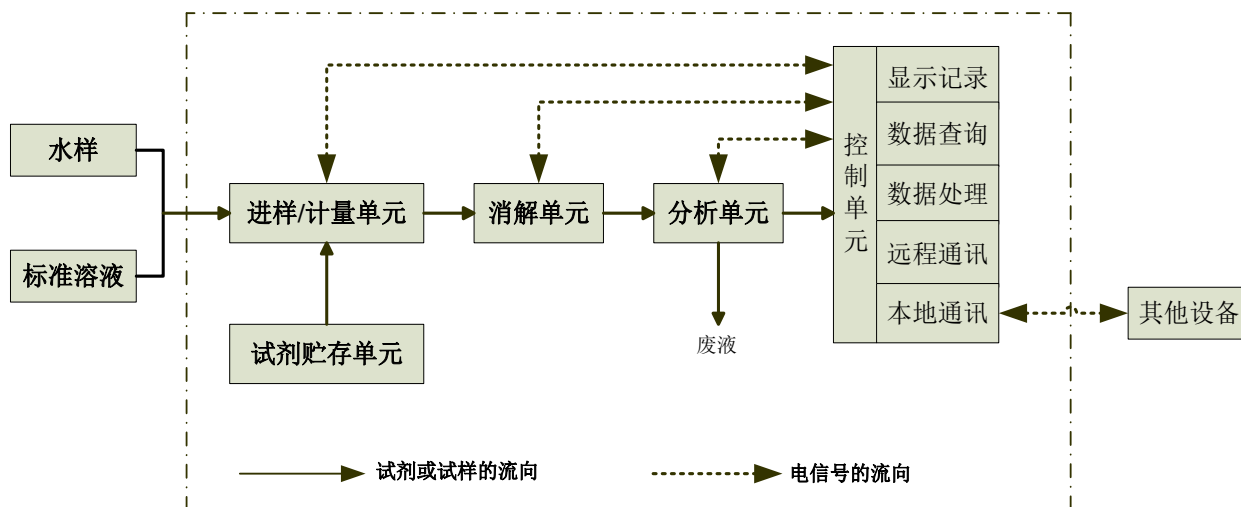
图 1 仪器的基本组成单元
