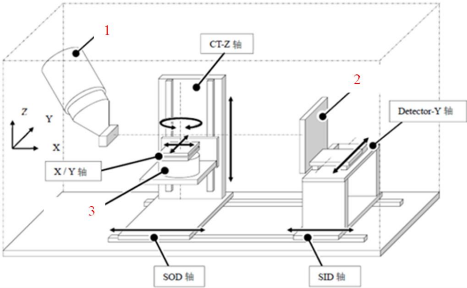
图 9-2 工业 CT 内部结构图
