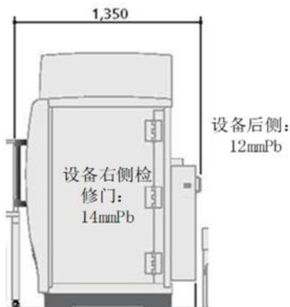
图 10-2 工业 CT 右视图（图中标注尺寸单位为 mm）
