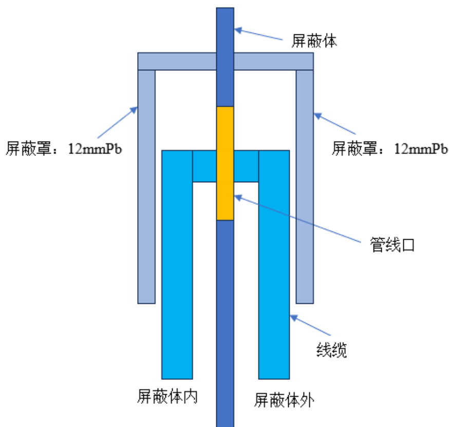
图 10-3 管线口屏蔽示意图
