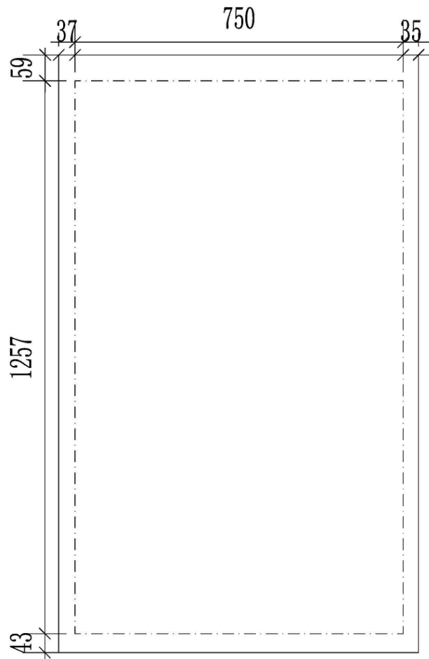
图 10-4 右侧检修门搭接示意图（单位：mm）
