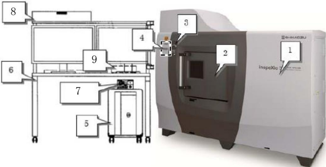
图 9-1 工业 CT 外观结构图
