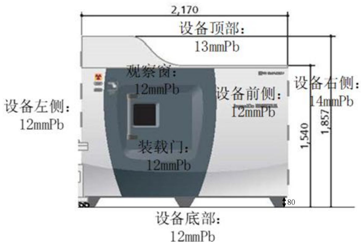
图 10-1 工业 CT 主视图（图中标注尺寸单位为 mm）
