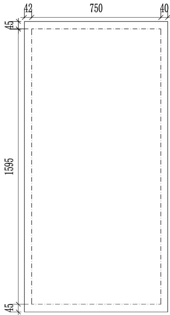
图 10-5 左侧检修门搭接示意图（单位：mm）
