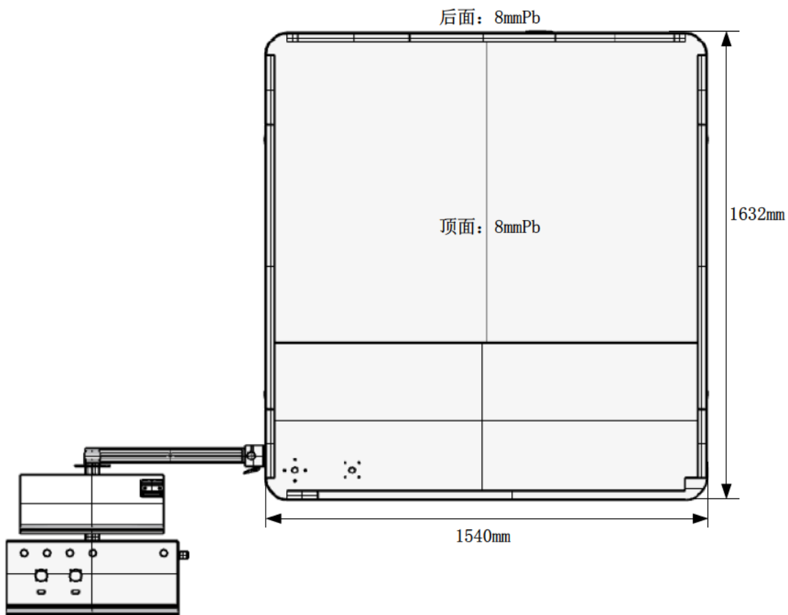
图 10-2 工业 CT 俯视图
