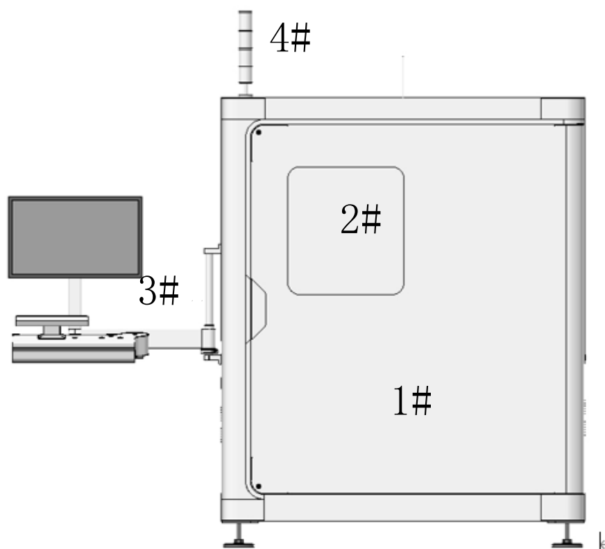
图 9-1 工业 CT 外观结构图
