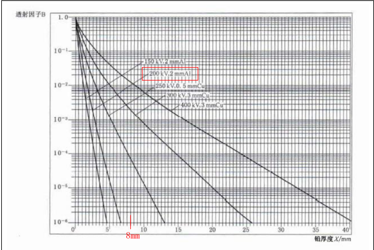
图 11-3 X 射线穿过铅的透射因子
