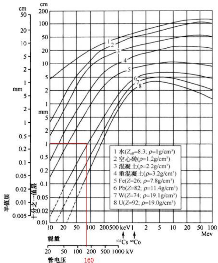
图 11-4 屏蔽材料的平衡十分之一值层
