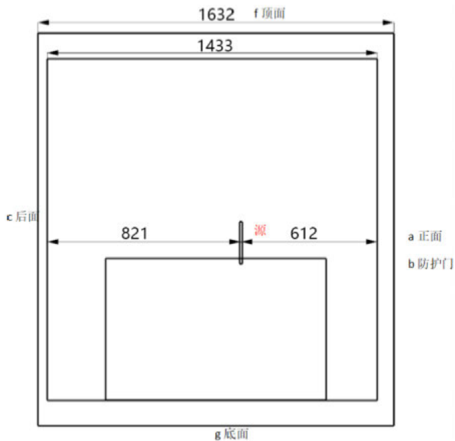
图 11-1.2 射线源分布示意图（俯视图，图中标注尺寸单位为 mm）
