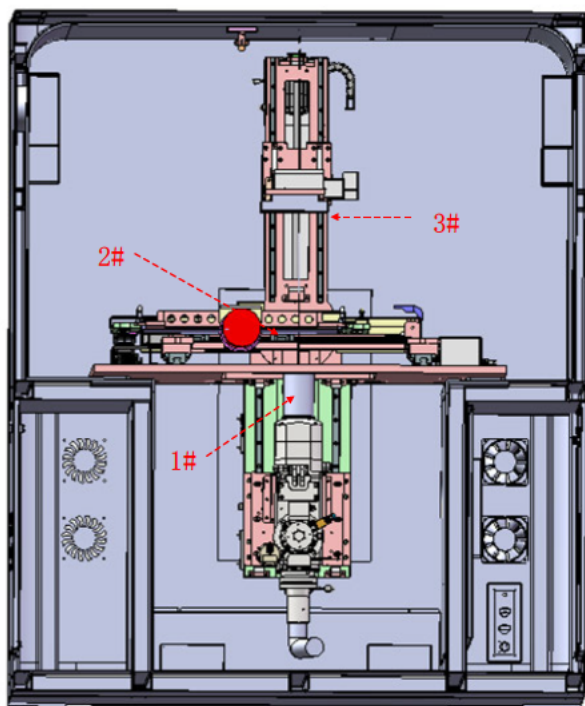
图 9-2 工业 CT 内部结构图
