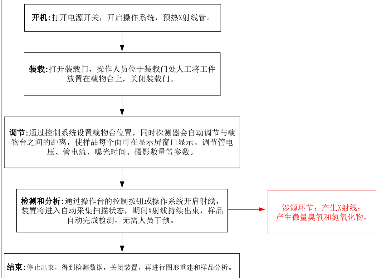
图 9-5 工艺流程和产污环节图
