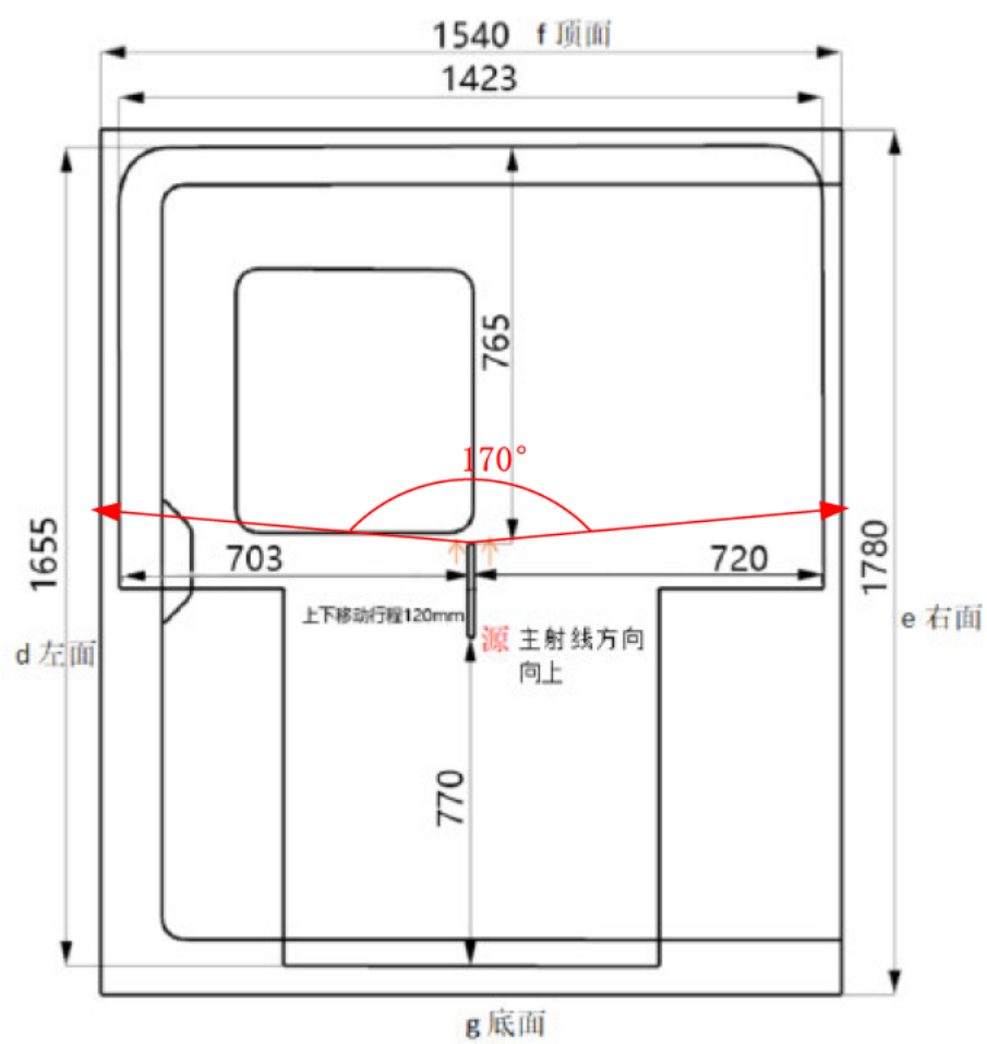
图 11-1.1 射线源分布示意图（主视图，图中标注尺寸单位为 mm）
