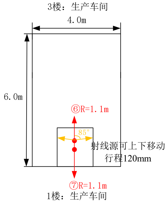
图 11-2.2 关注点分布示意图（立面）
