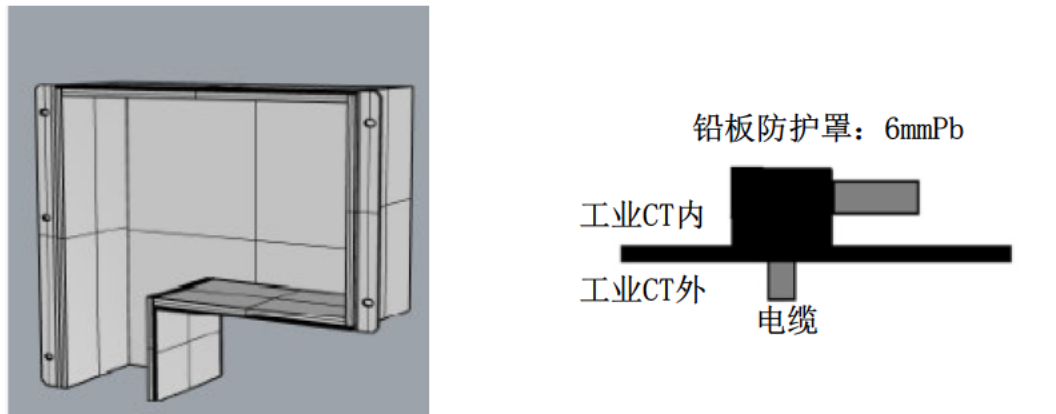
图 10-3 管线穿屏蔽体示意图
