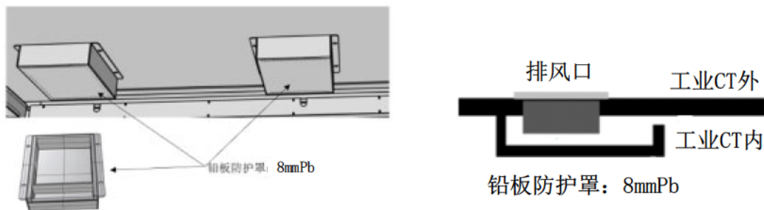
图 10-4 排风口屏蔽示意图
