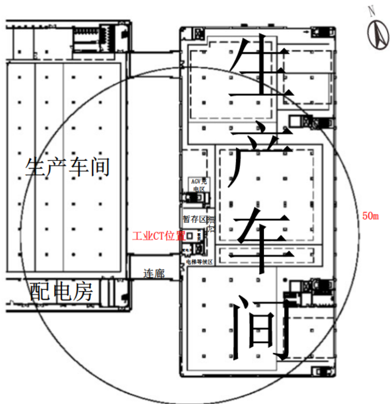
图 1-3 三号厂房 2 楼平面布置图
